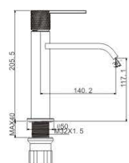
MI1633-827LSJ Basin faucet
