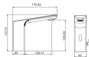
SF11017HCP-A Sensor faucet
