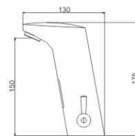
SF11003HCP-A Sensor faucet
