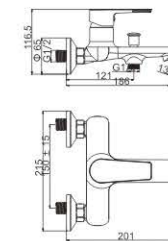
M31534-200C Bath faucet
